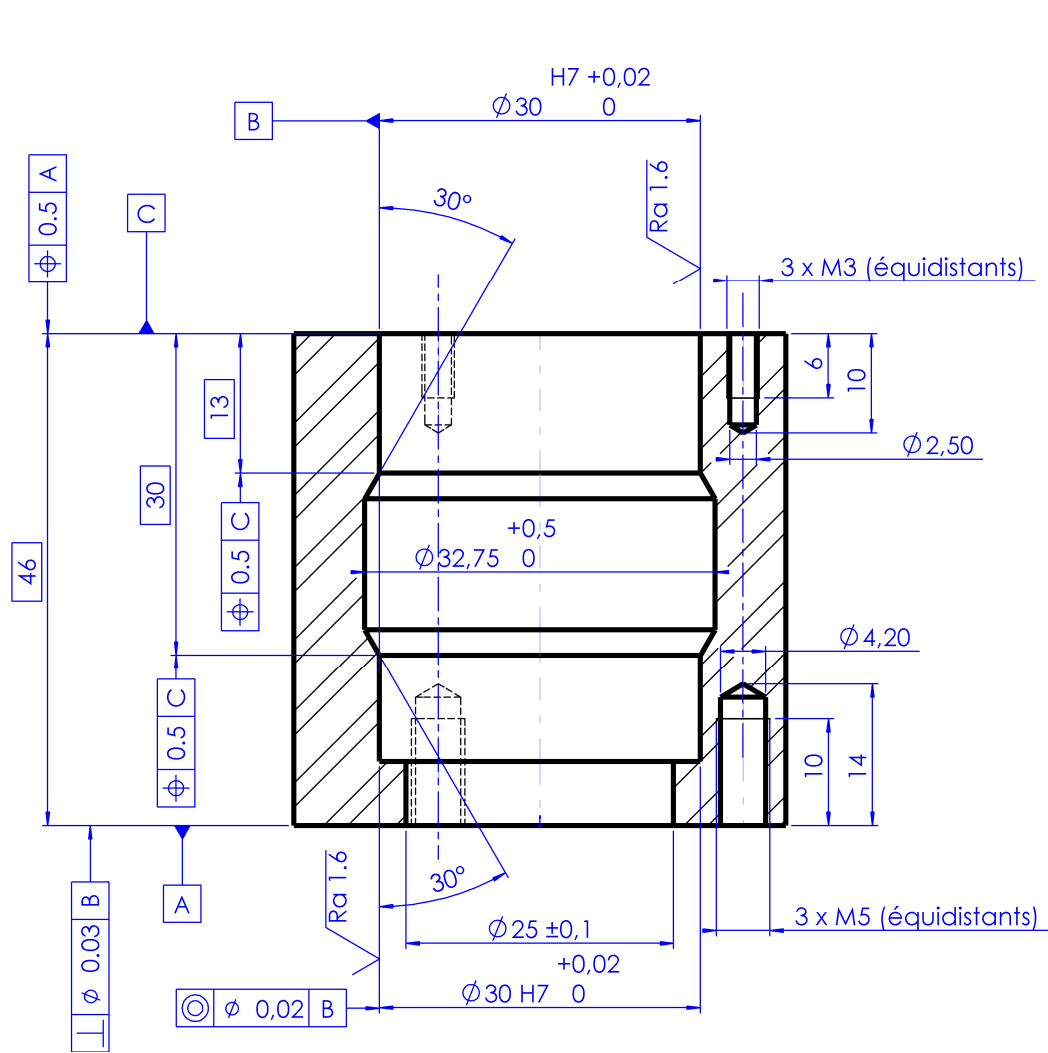
COUPE A-A ECHELLE 2 : 1
